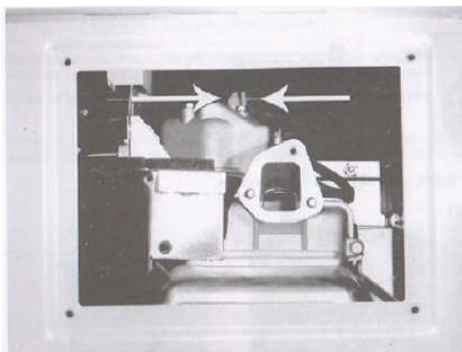
Figura A – Scoateți panoul lateral, apoi scoateți filtrul de aer. Căutați Maneta de decompresie „rosie” (în imaginea de mai sus este în poziția SUS). Apăsați maneta în jos – acest lucru va duce la deschiderea supapei de eșapament. Puneți la loc ansamblul cu filtrul de aer. Porniți motorul. Veți vedea că maneta cu arc va reveni automat la poziția SUS (UP). (Denumiți și ansamblul de decompresie pe unele scheme.)
